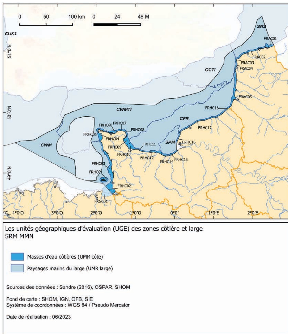
Figure 1 : Cartographie des différentes unités géographiques d'évaluation (masses d'eau côtières de la Directive Cadre sur l'Eau et paysages marins OSPAR) de la sous-région Marine Manche- Mer du Nord. SNS : Southern North Sea ; CCTI : Channel coastal shelf tidal influenced; CFR : Coastal FR channel; SPM : Seine plume ; CWMTI : Channel well mixed tidal influenced ; CWM : Channel well mixed.
