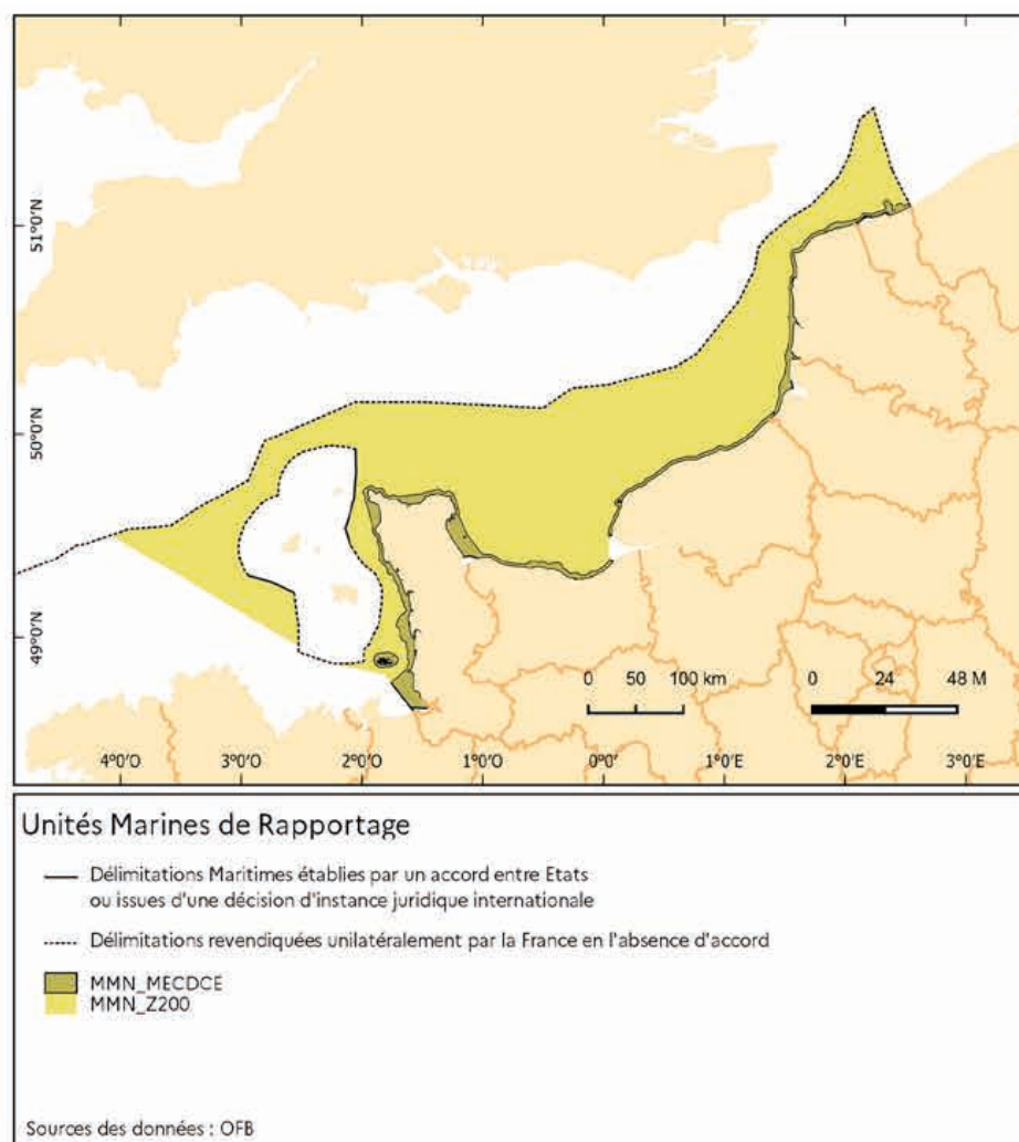
Figure 1 : Unités marines de rapportage pour la sous-région marine Manche - Mer du Nord. Emprise des Masses d'Eau Côtières de la Directive Cadre sur l'Eau (MECDCE) et zone du plateau allant jusqu'à la limite des 200 mètres de bathymétrie (Z200).
