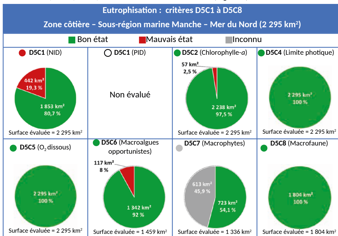
Figure 5 : Evaluation des différents critères du descripteur 5 pour la zone côtière de la sous-région marine Manche - Mer du Nord. Etat du critère bon / mauvais / inconnu ; surface (km 2 ) et proportion (%) de surface évaluée pour les différentes classes d'état du critère. Les masses d'eau côtières DCE pour lesquelles aucune évaluation n'est renseignée ne sont pas représentées.
