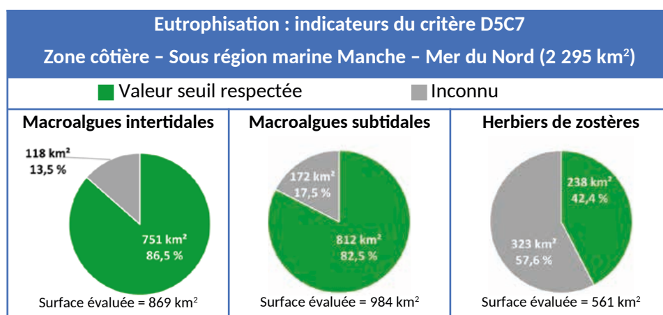
Figure 4 : Evaluation des trois indicateurs renseignant le critère D5C7 pour la zone côtière de la sous-région marine Manche - Mer du Nord : surface (km²) et proportion de la surface évaluée (%) pour laquelle la valeur seuil est bien respectée (vert) ou aucune évaluation n'est possible (gris).
