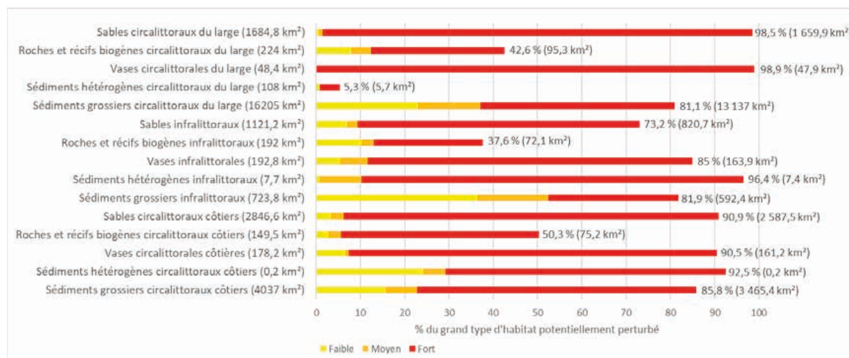
Figure 7 : Proportion (%) et étendue (km²) des grands types d'habitats soumis à risque d'effets néfastes (en lien avec l'abrasion) dans la sous-région marine Manche - Mer du Nord. En jaune : risque faible ; en orange : risque moyen ; en rouge : risque fort. Les deux grands types d'habitats benthiques intertidaux sont dans un état inconnu.
