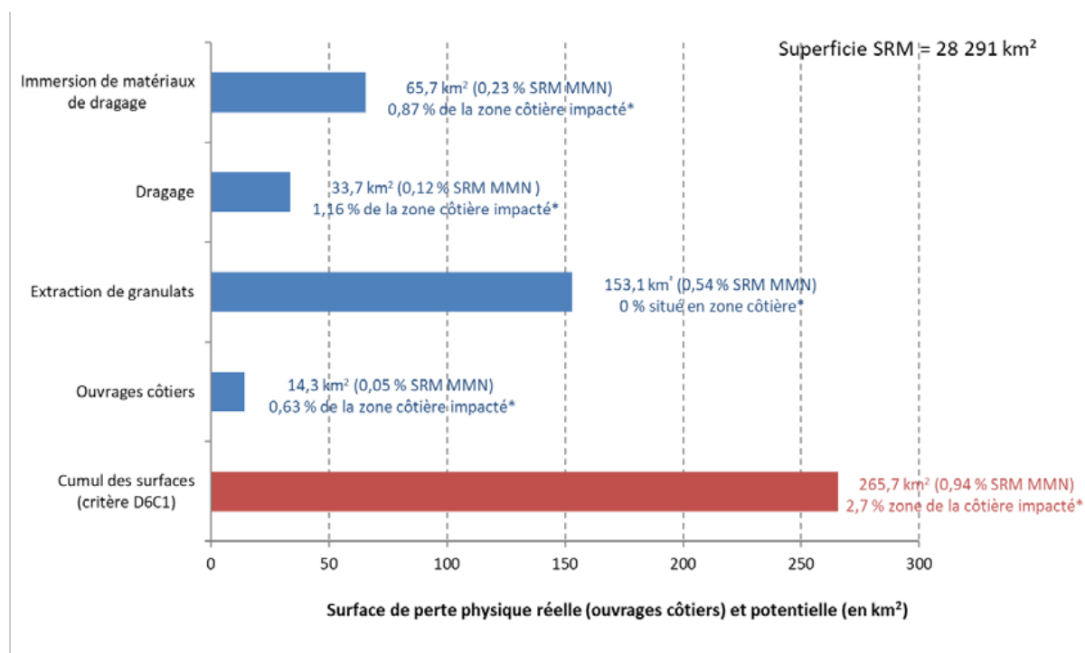
Figure 2 : Etendue spatiale (en km 2 et en % de surface de la sous-région marine Manche - Mer du Nord) de la perte physique due à chacune des activités considérées pour l'évaluation du critère D6C1 (en bleu) et cumul surfacique à l'échelle du critère (en rouge). * A titre illustratif, le pourcentage de la surface de la zone côtière subissant des pertes physiques induites par chacune des activités est également présenté.
